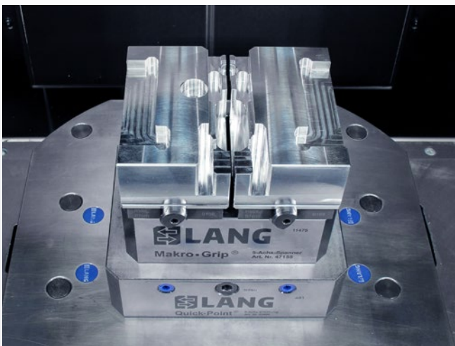
Avanti 125 Konturspanner mit Aluminium Aufsatzbacken. Bild: Thoma Tec.
