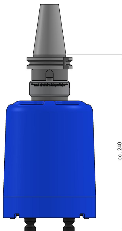
Spannmittelhaube mit SK 40
